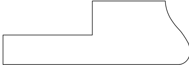
TRIM141 1 1/16" x 3 3/16"
